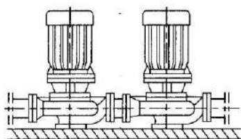
多段横式配装
