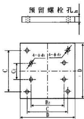
联接板
