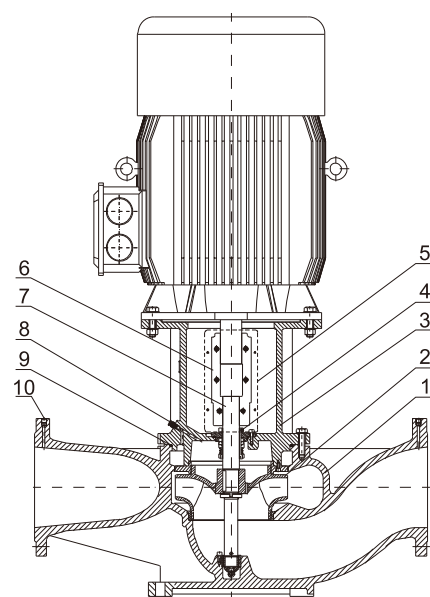
TD200-TD250 材料表
