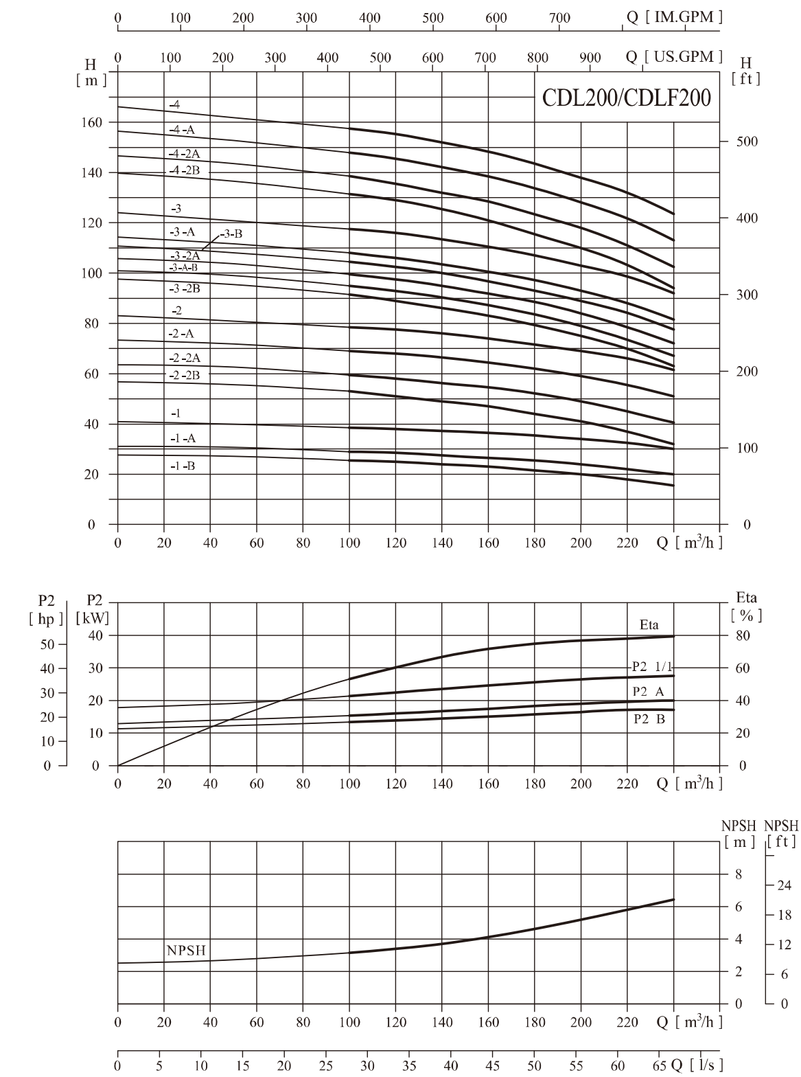
性能曲线
