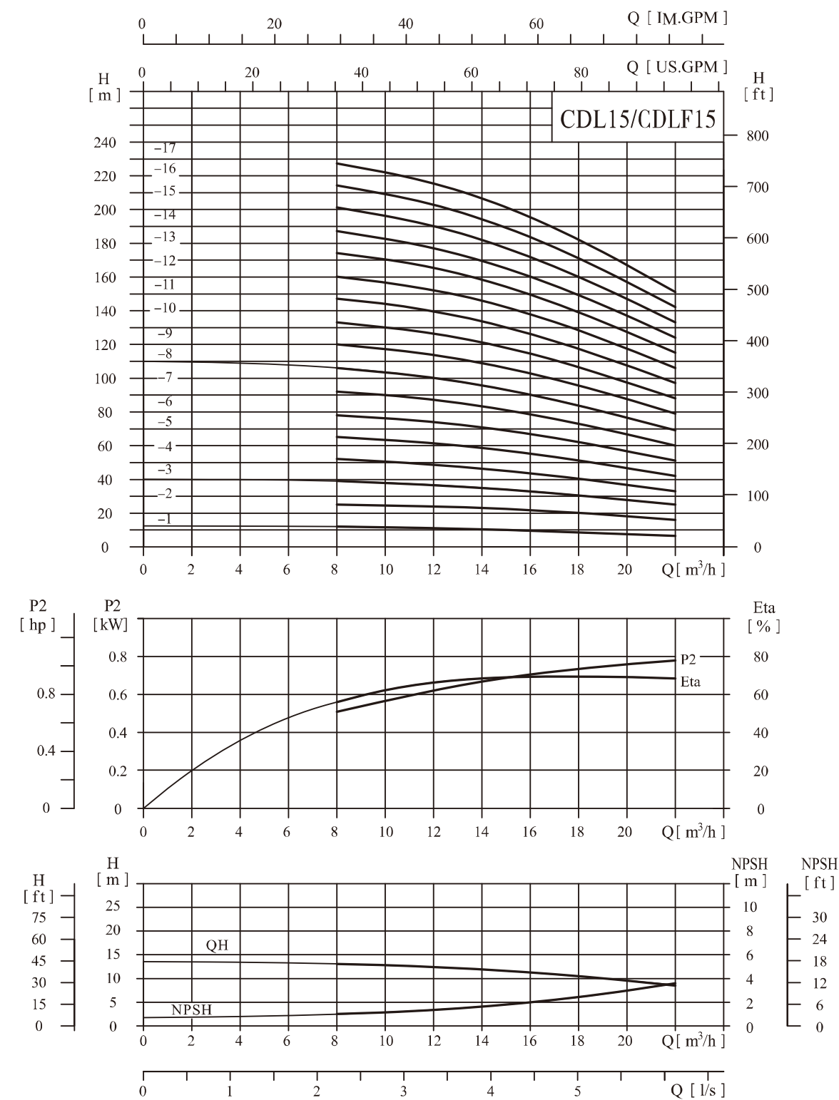
性能曲线
