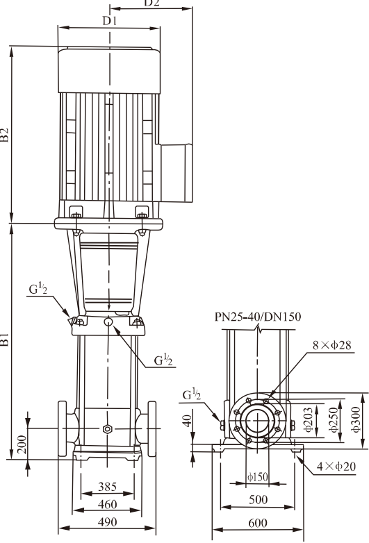
安装图
