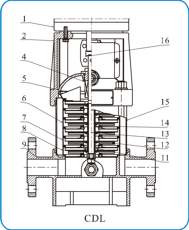
截面图 CDL,CDLF 2,4
