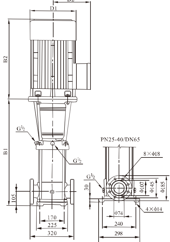
安装图
