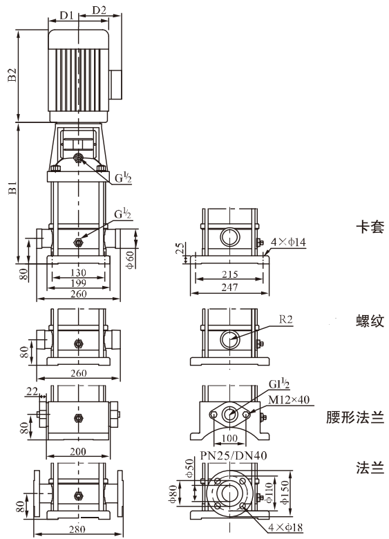
安装图
