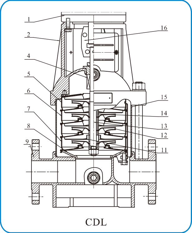
截面图 CDL,CDLF8,10,12,15,20
