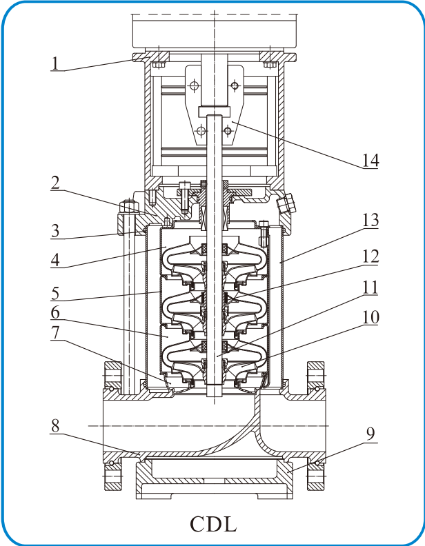
截面图 CDL,CDLF32,42,65,85
