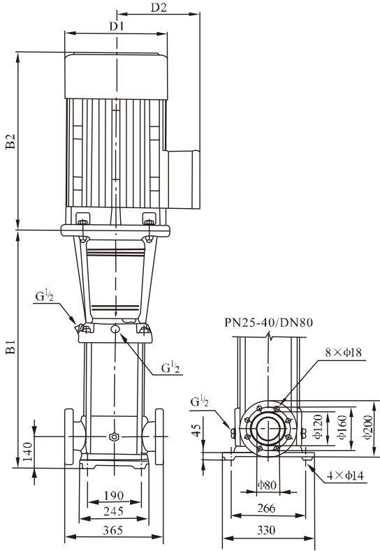
安装图
